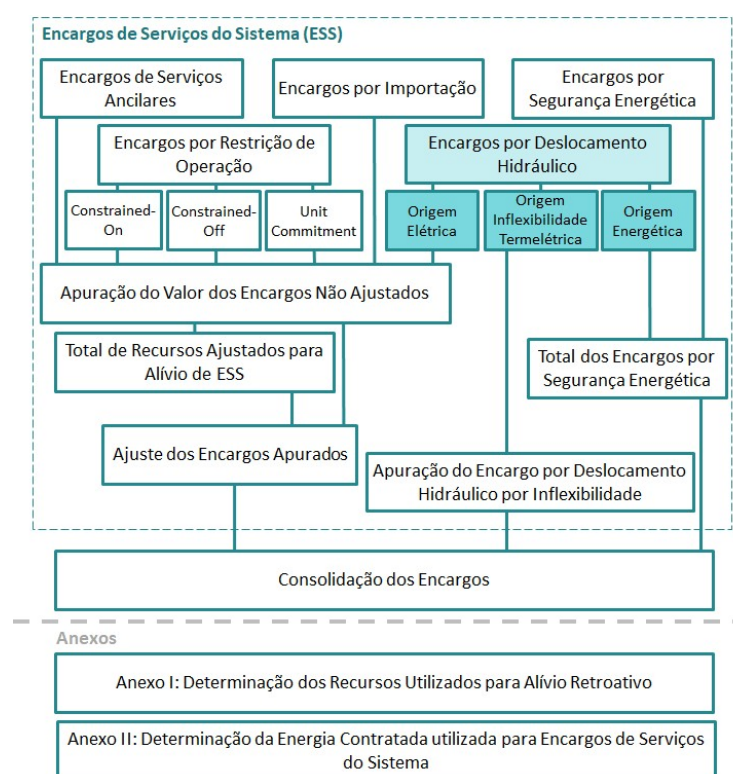
Figura 14: Esquema Geral do Módulo de Regras: “Encargos”
